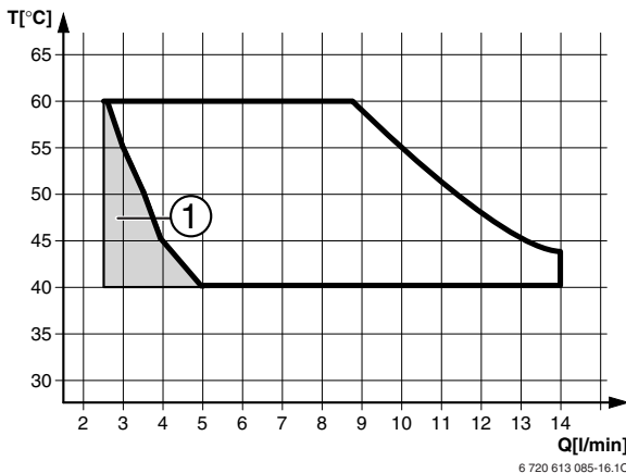
Res. 11 Sıcak Kul. Suyu Performans Diyagramı (Giriş Suyu Sıcaklığı = +15 °C) (B1 RDW 28 81 / ZWC 28-3..)
