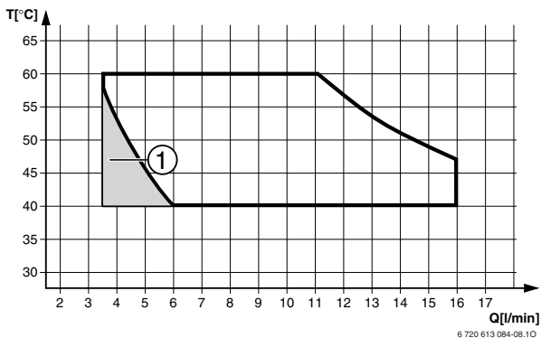
Res. 12 Sıcak Kul. Suyu Performans Diyagramı (Giriş Suyu Sıcaklığı = +15 °C) (B1 RDW 35 81 / ZWC 35-3..)
